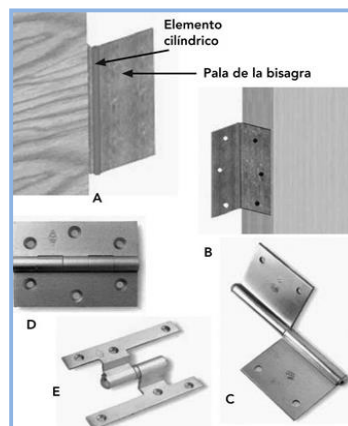
Fig. 15 Diferentes dispositivos de giro aplicable a puertas y ventanas, bisagra pomel A y B, de clavija C, bisagra corriente con pasador incorporado D y bisagra en H, con pasador menor que las palas, que permite que quede un mayor distanciamiento entre el marco y la hoja de la puerta.
