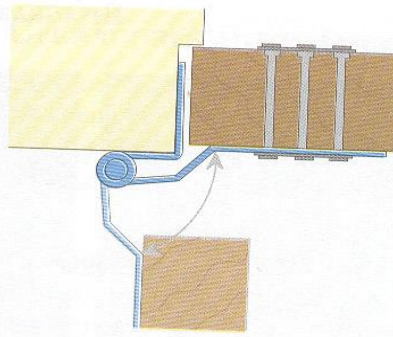
BISAGRA DE VIAJE DE MEDIA SUPERFICIE
