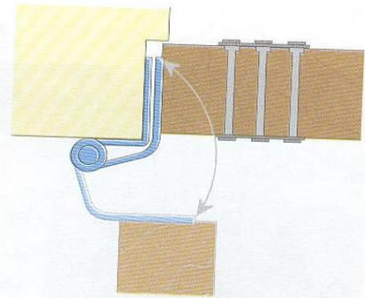
BISAGRA DE VIAJE EMBUTIDA
