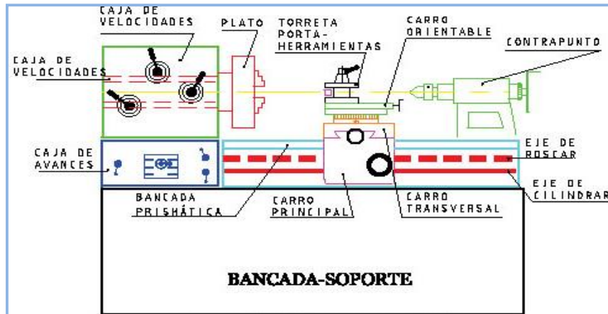
Fig. 17 Esquema de torno paralelo.
