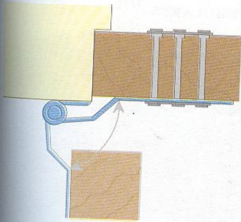
BISAGRA DE VIAJE DE SUPERFICIE COMPLETA
