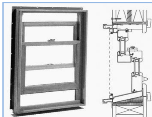
Fig. 1.26 Ventana de guillotina.
