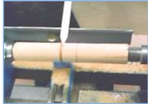
Figs. 73 y 74 Trazo y corte oblicuo.
